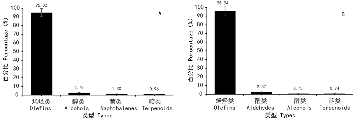
图 2 资源冷杉(A)与元宝山冷杉(B)针叶精油化学组分
