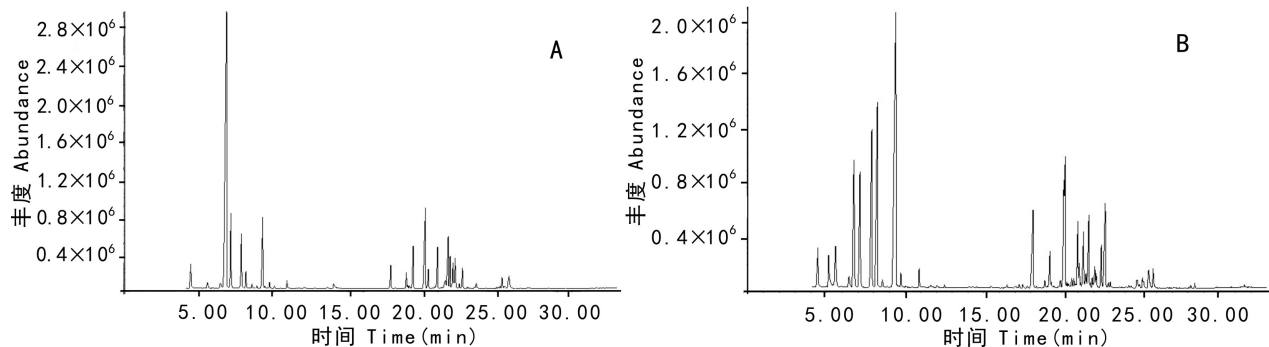
图 1 资源冷杉(A)和元宝山冷杉(B)针叶精油总离子流图
