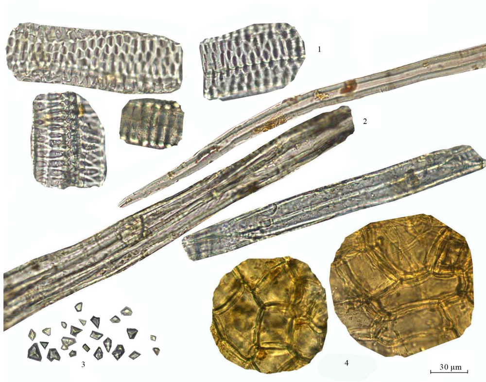
1. 导管; 2. 纤维; 3. 草酸钙砂晶; 4. 木栓细胞。 1. Vessel; 2. Fiber; 3. Calcium oxalate sand crystal; 4. Phellem cell.
