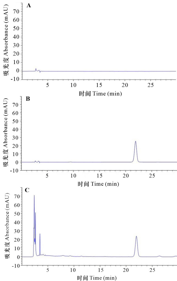
图6 空白溶剂(A)、 \beta -蜕皮甾酮对照品(B)和供试品(C) HPLC 色谱图
