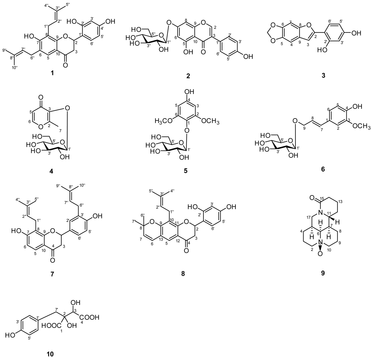
图 1 化合物 1-10 的结构式 Fig. 1 Structures of compounds 1-10
