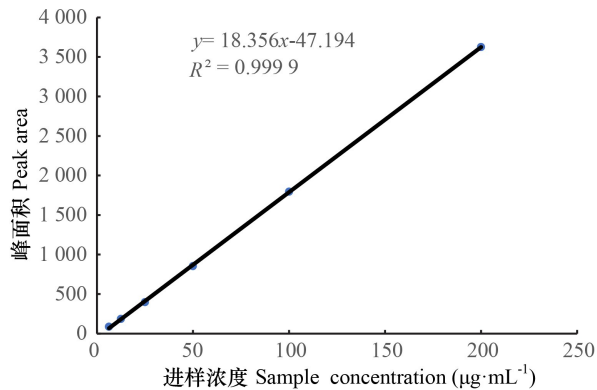
图 5 广藿香酮线性关系图
