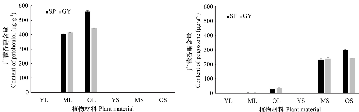
图7 石牌广藿香和高要广藿香栽培种广藿香醇和广藿香酮的含量
