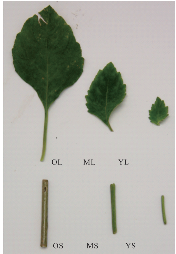
OL. 老叶; ML. 成熟叶; YL. 幼叶; OS. 老茎; MS. 成熟茎; YS. 幼茎。下同。
