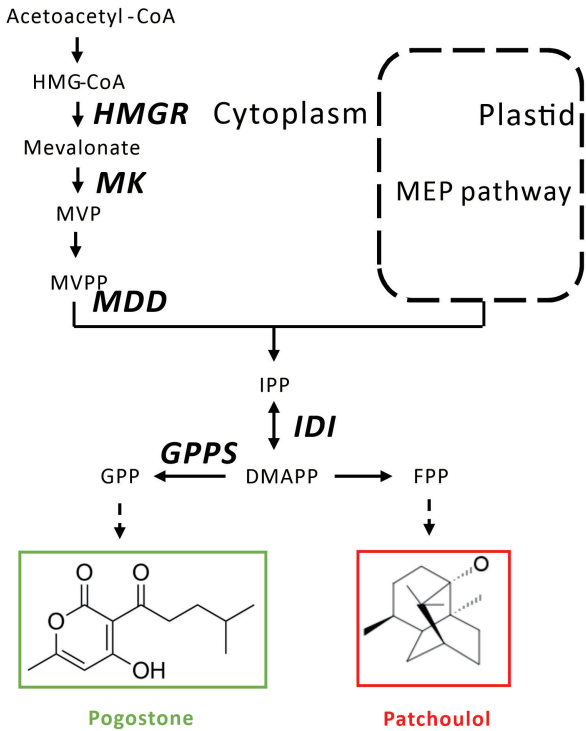
图 1 MVA 萜类代谢途径相关基因
