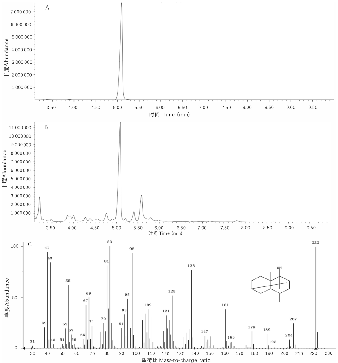
A. 广藿香醇标准品总离子色谱图; B. 广藿香醇挥发油总离子色谱图; C. 广藿香醇质谱图。
