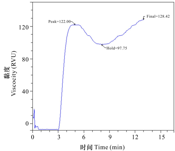
图6 食用观音座莲蕨粉的糊化特性曲线
