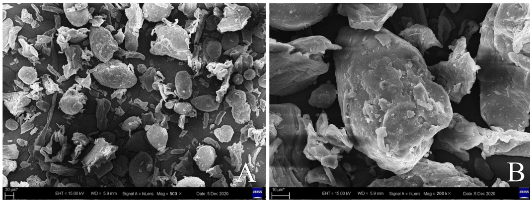
图 2 食用观音座莲蕨粉颗粒的扫描电镜图 (A) (放大倍数为 500 ×) 和食用观音座莲蕨粉颗粒的扫描电镜图 (B) (放大倍数为 200 k ×)
