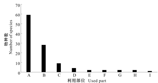
图 3 白裤瑶猪饲料植物的利用部位统计 Fig. 3 Statistics for used parts of Baiku Yao forage plants
